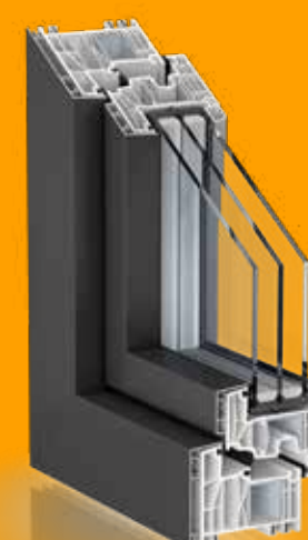
AluClip Plus
